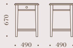
2. Rebecca naktskapis
